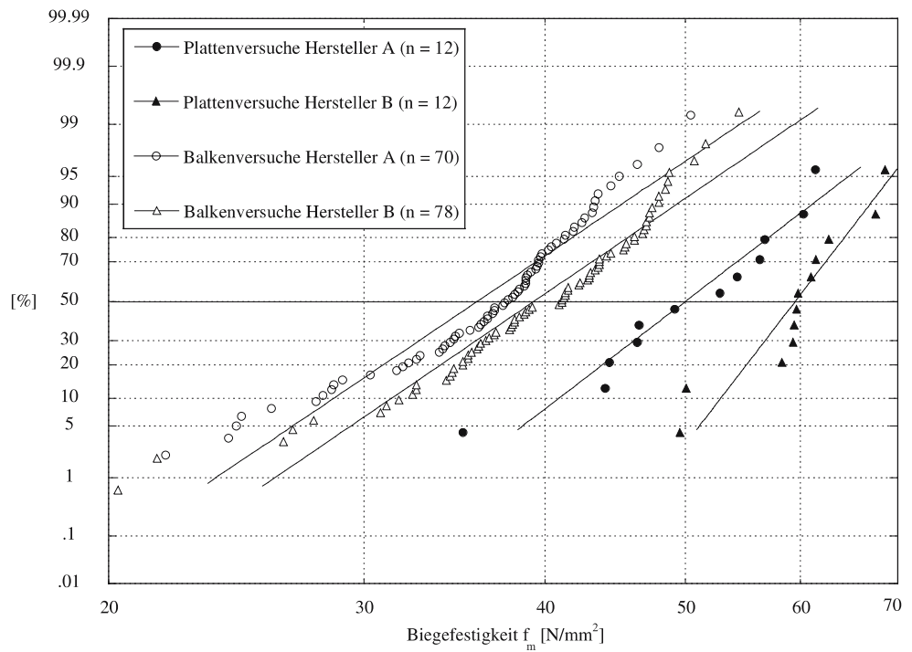
Abb. 9 Vergleich der Biegegrandspannungen bei Bruchlast ermittelt aus den Versuchen an Balken und an Platten Fig. 9 Comparison of flexural stress at failure determined from beam and from panel tests
