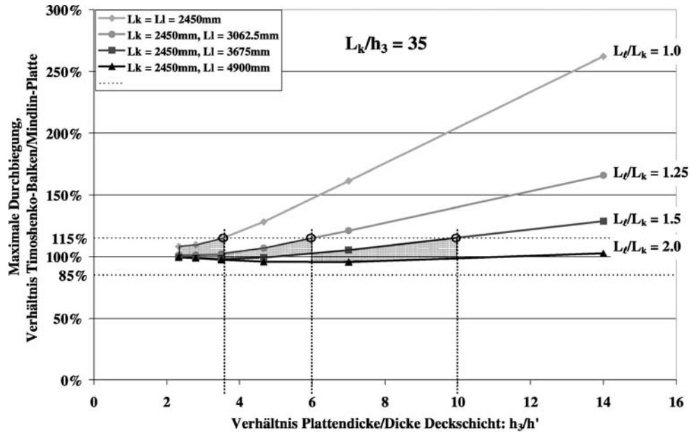
Abb. 14 Vergleich der berechneten Durchbiegung für verschiedene Plattenaufbauten: Timoshenko-Balken (mit Schubverformung) und Mindlin–Reissner-Platte (mit Schubverformung und Plattentragwirkung) Fig. 14 Comparison of the calculated deflections for different plate compositions: Timoshenko-Beam (with shear deformation) and Mindlin–Reissner-Plate (with shear deflection and plate load bearing behaviour)
