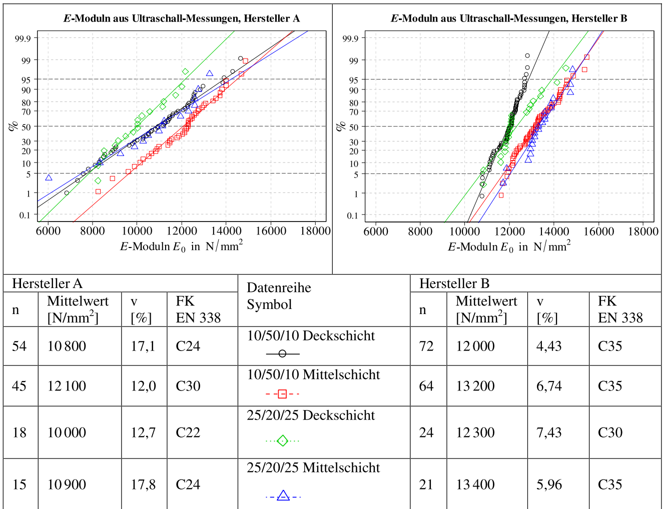
Abb. 5 Elastizitätsmodul der Einzelschichten bestimmt mittels Ultraschallmessungen Fig. 5 Elastic modulus of single layers derived from ultrasonic measurements
