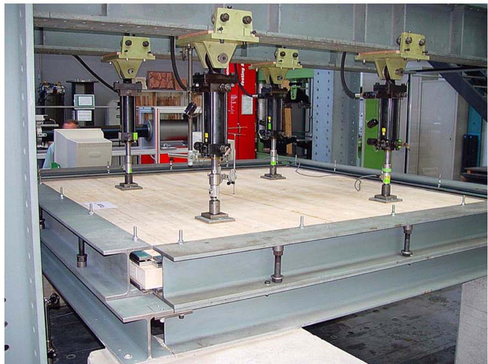
Abb. 3 Versuchseinrichtung mit allseitiger Linienlagerung, 4 Einzellasten Fig. 3 Test set-up with all-sided line support, 4 single loads
