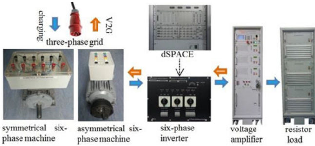
Fig. 9. Experimental rig.
