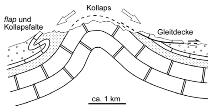
Kollaps Strukturen an den Schenkeln einer grossen Antiklinale nach Harrison & Falcon 1934 Geol. Mag. 71, 529-539
