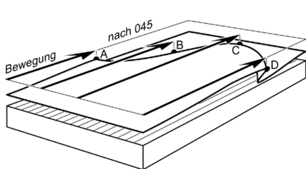
Kinematische Interpretation der nicht-zylindrischen Falten
