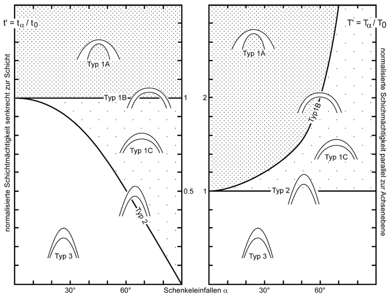
Morphologische Klassifikation basierend auf den Mächtigkeitsänderungen einer verfalteten Schicht nach Ramsay, 1967, McGraw-Hill Inc.
