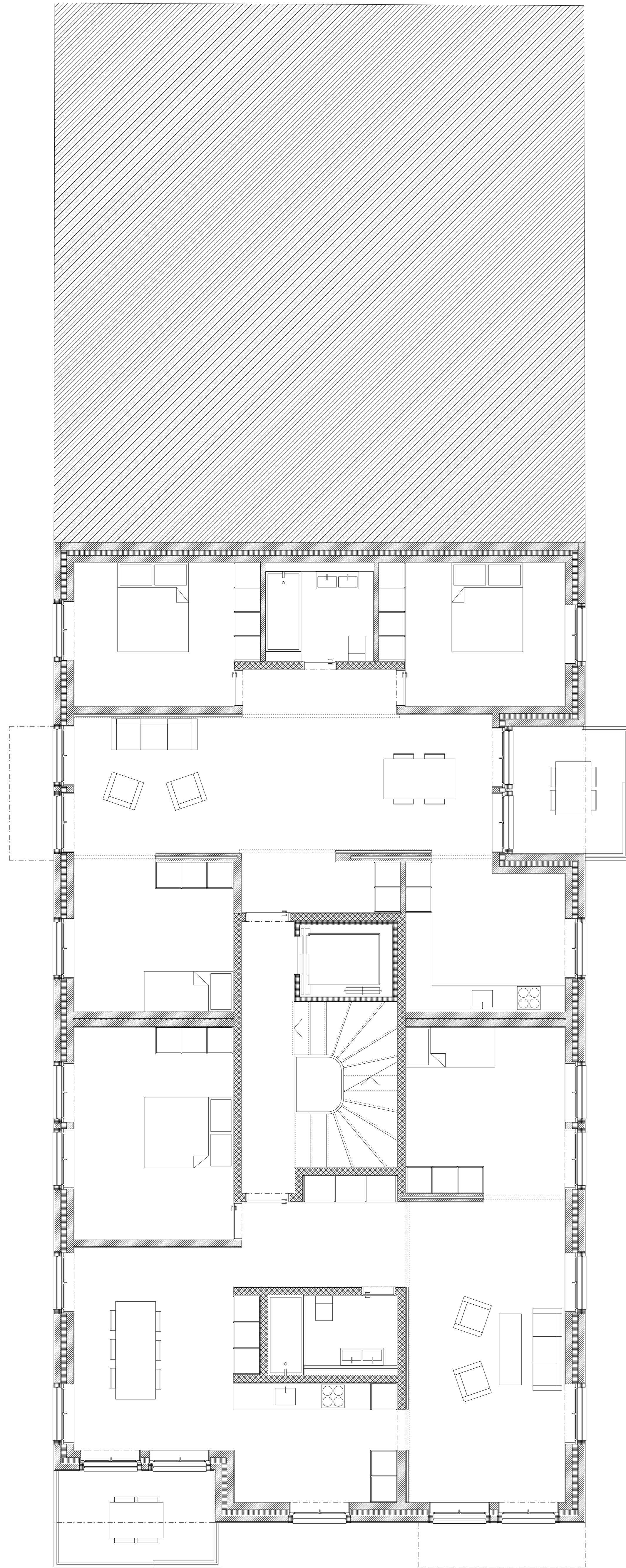
Erites / Drittes Obergeschoss 1:50
